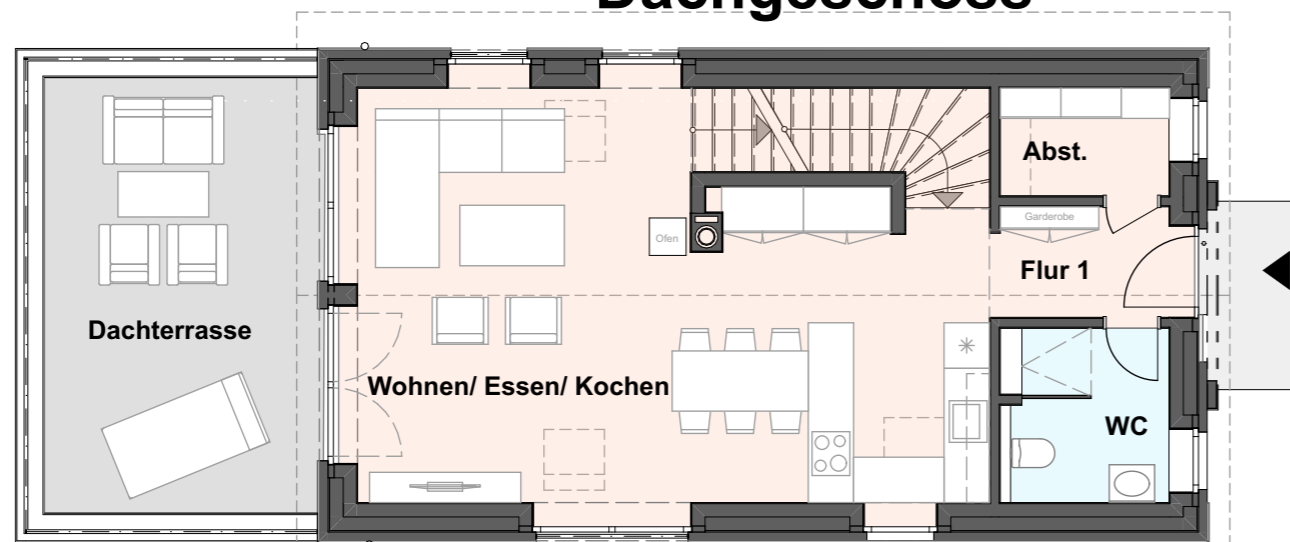
Erdgeschoss
