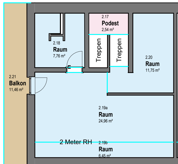
Dachgeschoss
