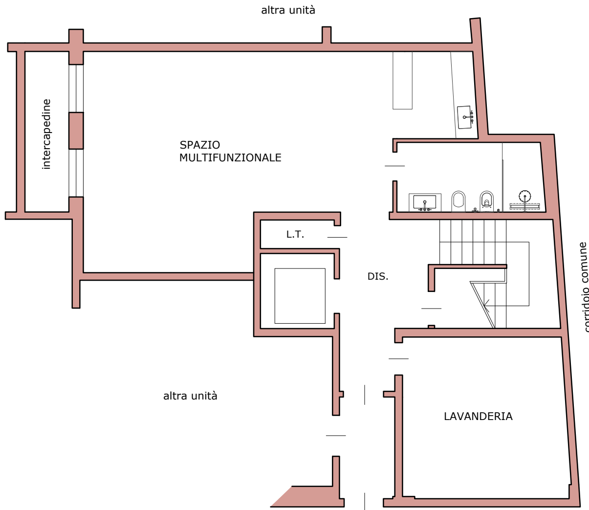
Piano Secondo Interrato H 2,69 m
