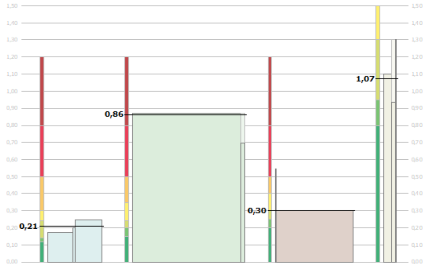
Flächenanteilige Aufteilung der Bauteil-U-Werte in W/m 2 K
